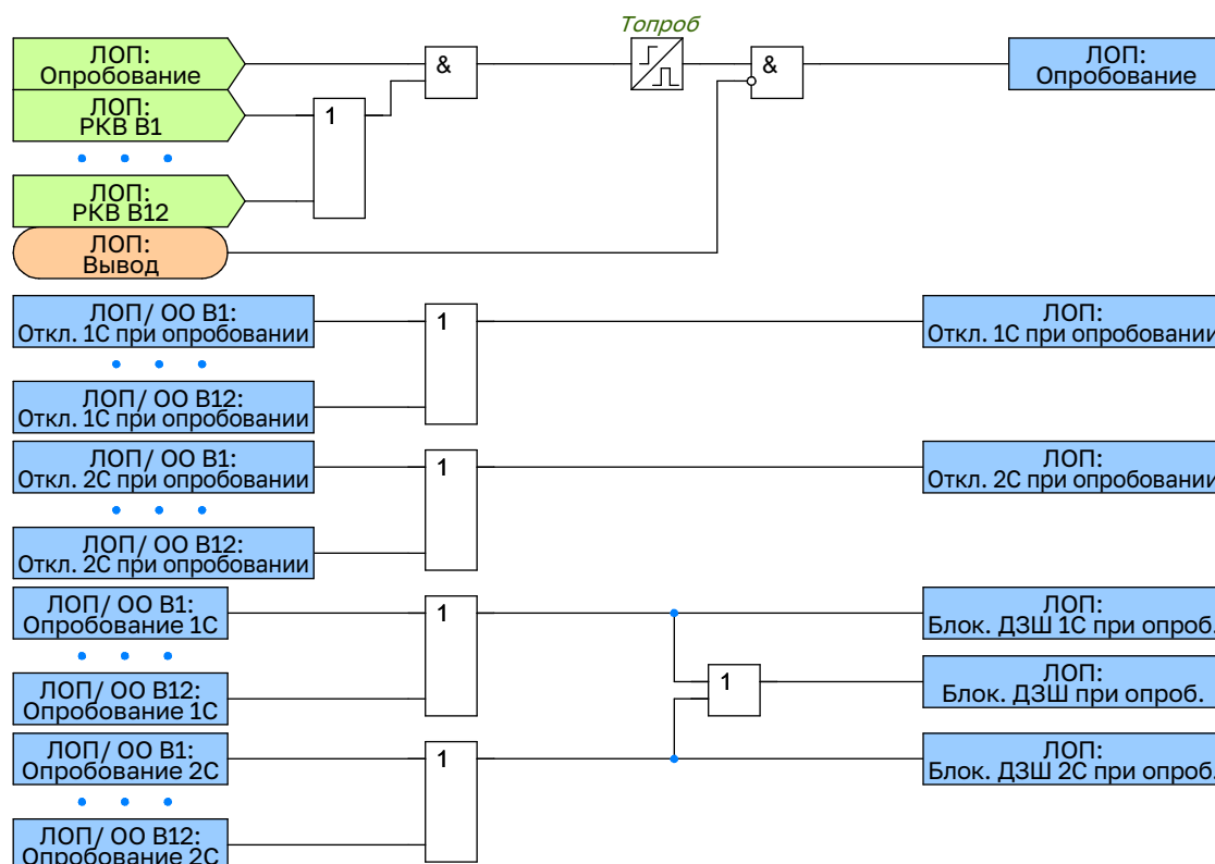
Рисунок 2.10 – Функциональная схема общей логики
